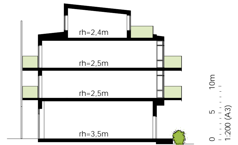
Sektion
